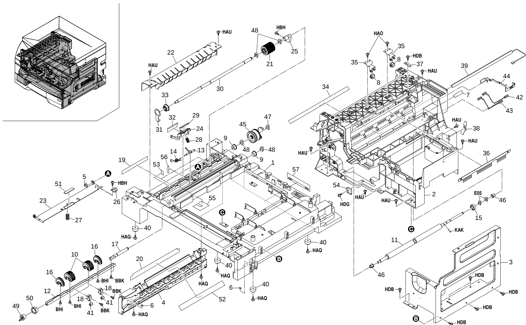
FIG. 2 FRAMES
